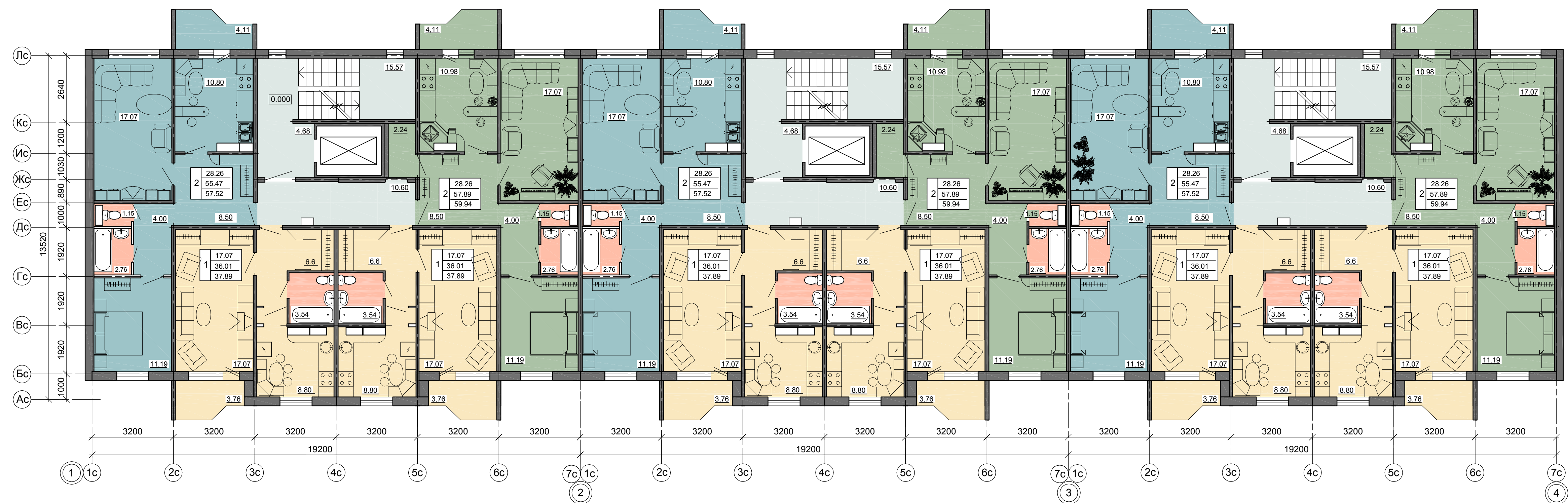
План типового этажа
